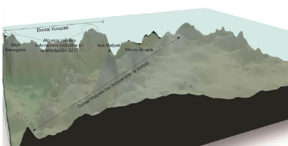
Figura 9. Modelación tridimensional de las dorsales Malpelo y Yuruparí, destacando algunos montes submarinos.
