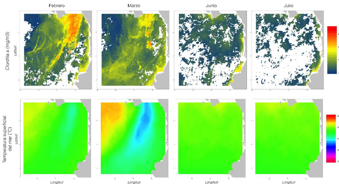
Figura 12. Productividad primaria (concentración de clorofila, arriba) y temperatura superficial del mar (grados centígrados, abajo) en la región del golfo de Panamá y la zona económica exclusiva de Colombia. Los datos corresponden a las condiciones oceanográfica. Tomado de: Bravo et al. (2021).
