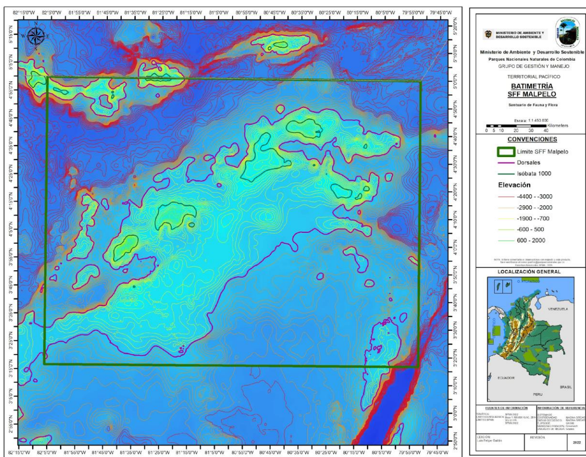
Figura 8. Batimetría de la cuenca central del pacifico con énfasis en la dorsal Malpelo y dorsal Yuruparí.
