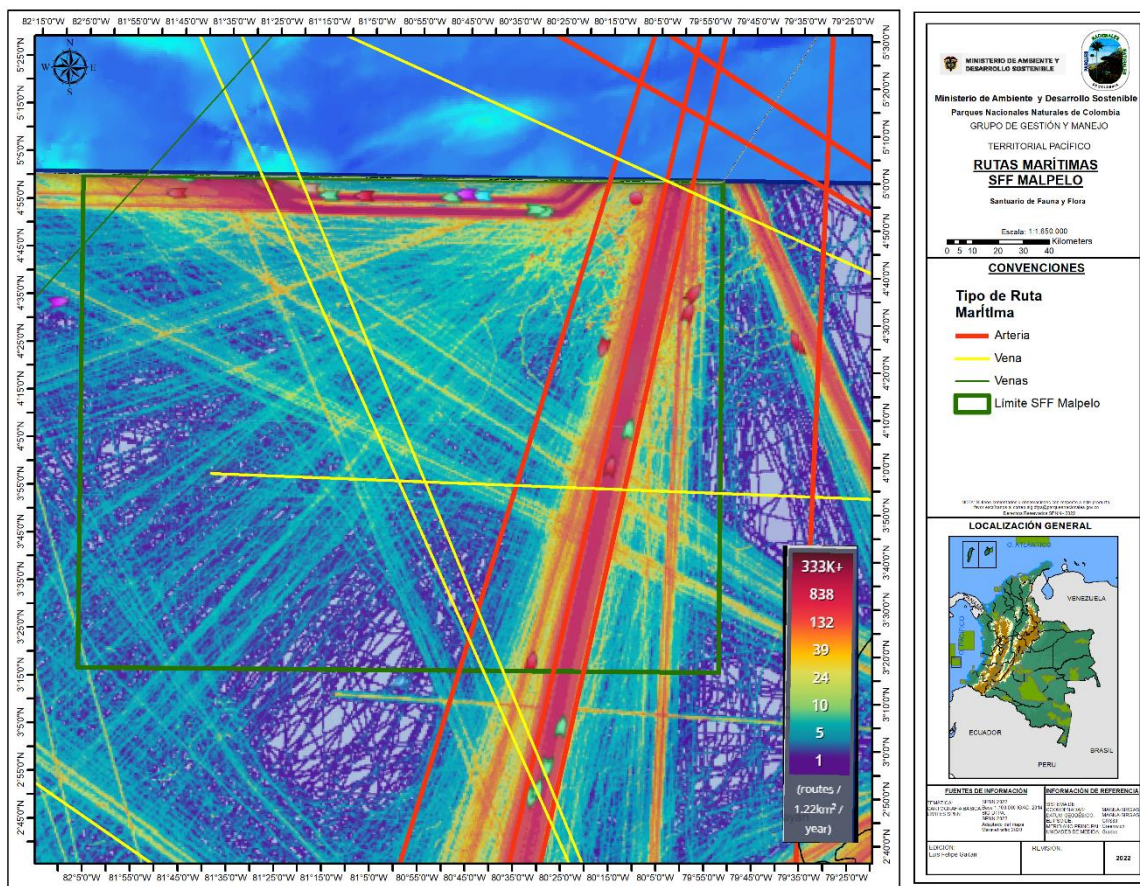
Figura 7. Principales rutas de los buques de tráfico internacional en el Pacífico Oriental.
