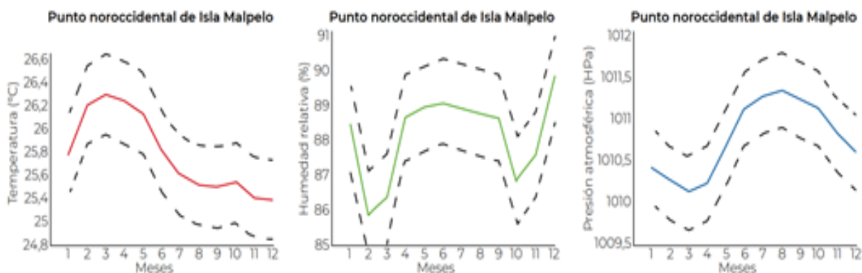
Figura 11. Comportamiento climático anual de la temperatura ambiente, humedad relativa y presión atmosférica, sobre Malpelo, representado con los promedios mensuales de estas variables desde 1958 hasta 2014. Tomado de: Niño et al. (2019).
